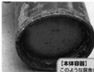
溶接部とその周辺の腐食
