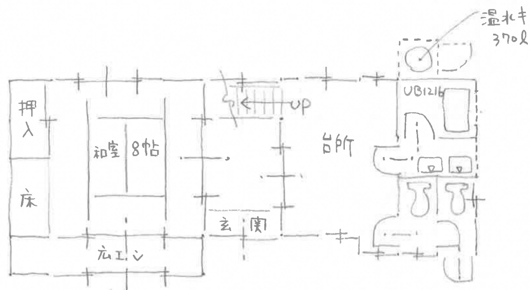
はなれ 1階平面図
