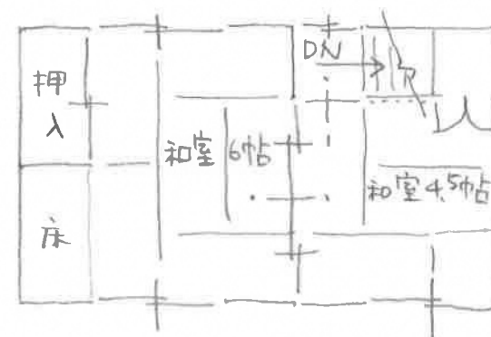
はなれ 2階平面図
